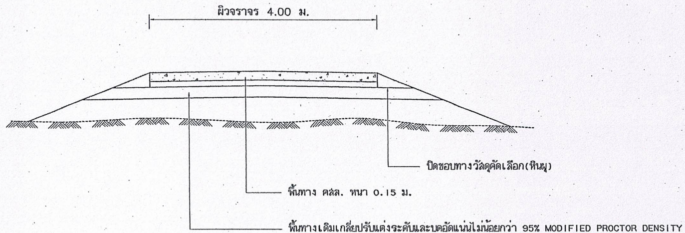
ภาพตัดตามขวาง
