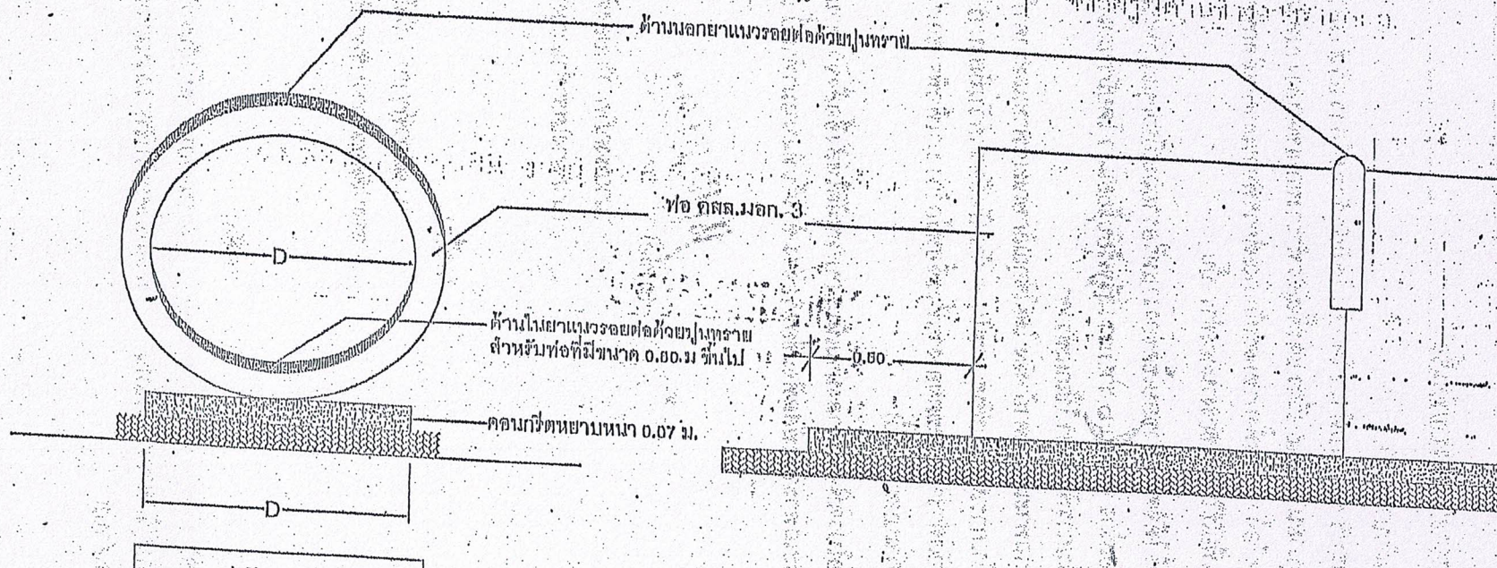
ขยายรูปตัดขวางท่อ คสล.
