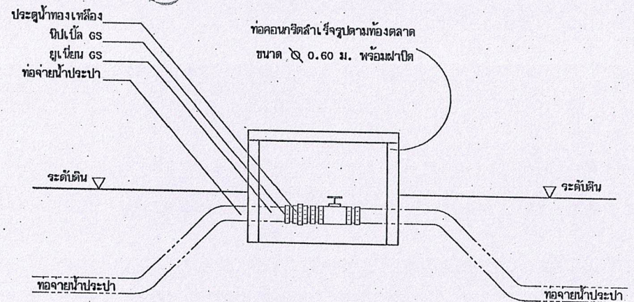
ขยายการติดตั้งประตุน้ำทองเหลือง
