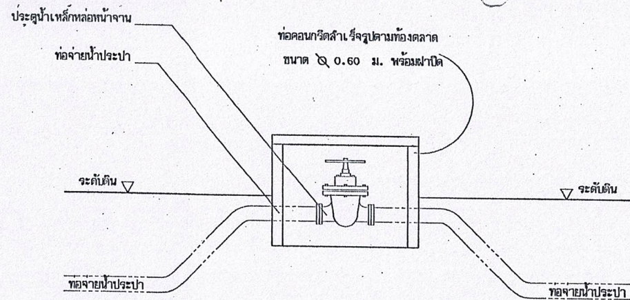
ขยายการติดตั้งประตุน้ำเหล็กหล่อ หน้างาน
