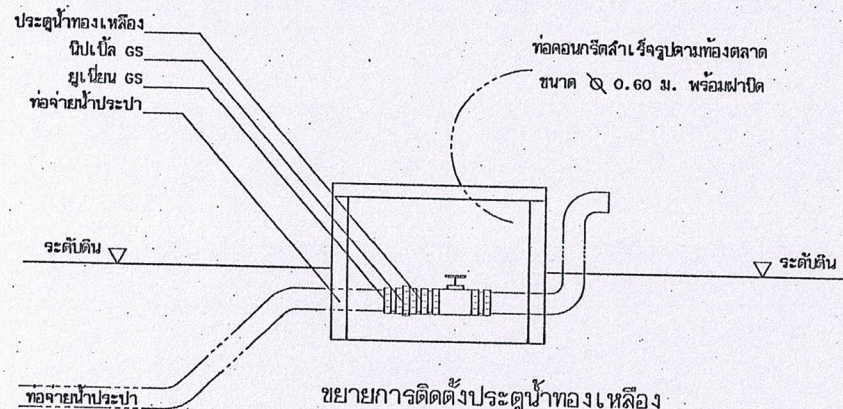
ขยายการติดตั้งประตุน้ำทองเหลือง จุดตามแนวท่อจ่ายน้ำ
