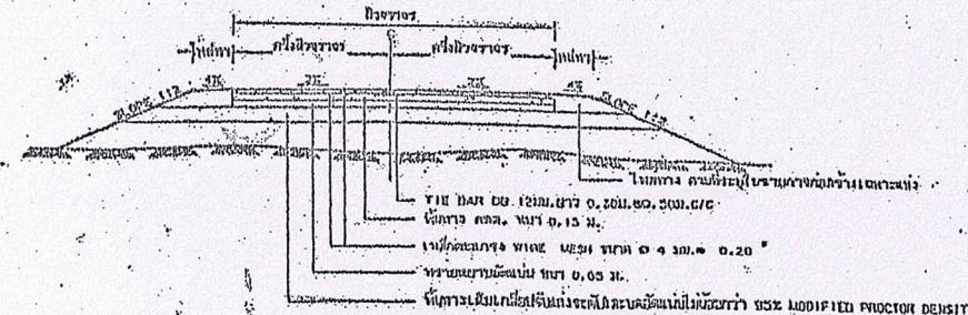
รูปตัดถนน คลส.
