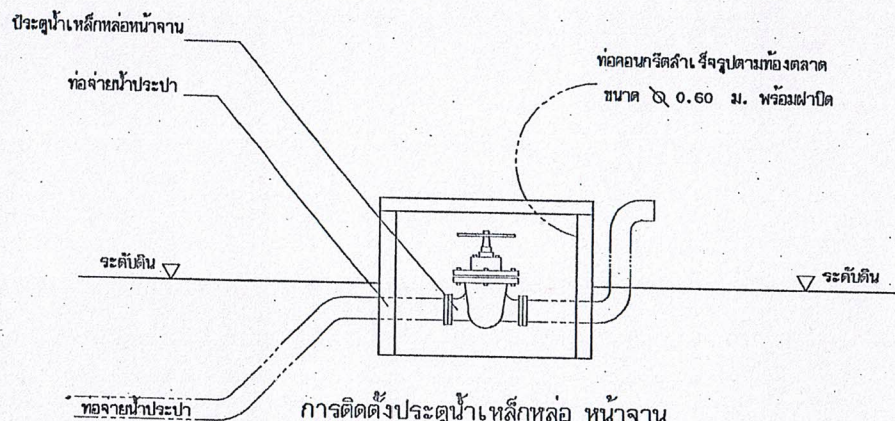
ขยายการติดตั้งประตุน้ำเหล็กหล่อ หน้างาน จุดตามแนวท่อจ่ายน้ำ
